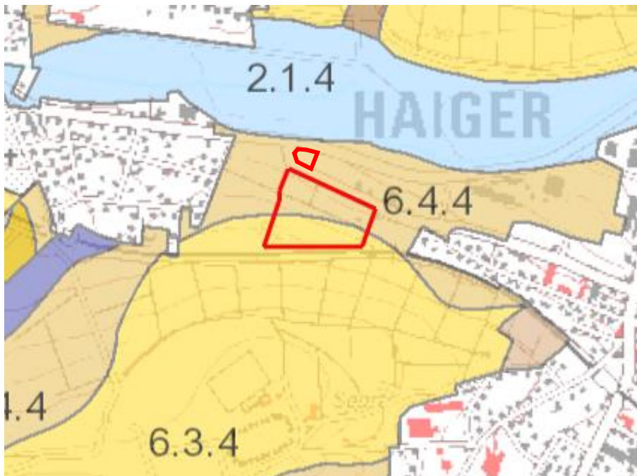
Abb. 7: Bodenhauptgruppen im Untersuchungsraum (HLNUG 2024-1).
